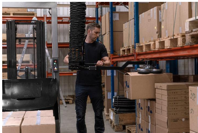
Mobiele orderpicker voor in het rek
